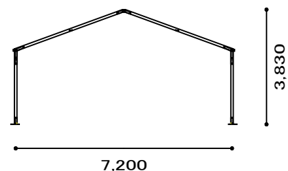
断面図(中間部)
