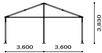
立面図
