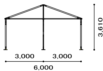
立面図
